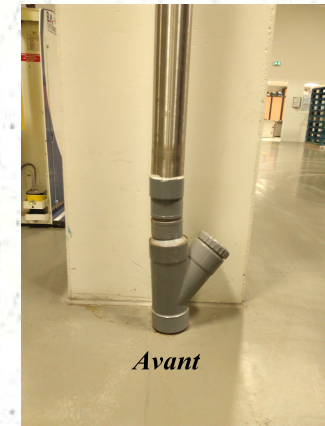
Modification écoulement PVC, par tuyauterie inox
